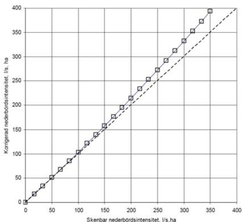
Figur 2-2 Exempel på effekten av korrigering av nederbörd tillämpad av Stockholm Vatten. Punkterna motsvarar nederbördsintensitet vid antalet vippningar per minut från 0 till 21 st. Streckad linje anger okorrigerade värden. Vippvolym 0,1 mm.
