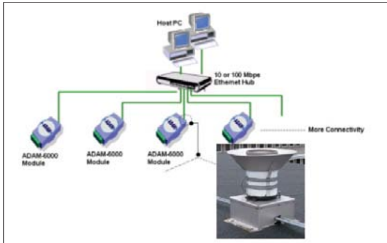
Figur 2-8 Princip för loggning av regnhändelser via nätverk
