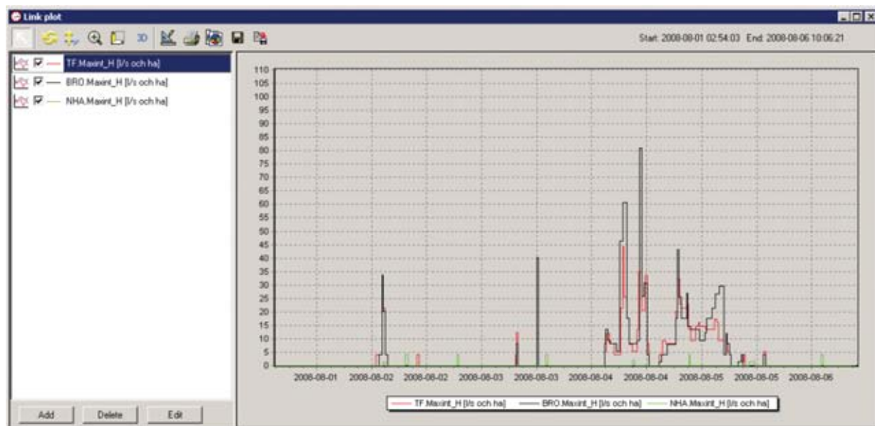
Figur 2-7 Exempel på översiktlig regnintensitetsbedömning i Helsingborg genom beräkning av flytande 10-minutervärde.
