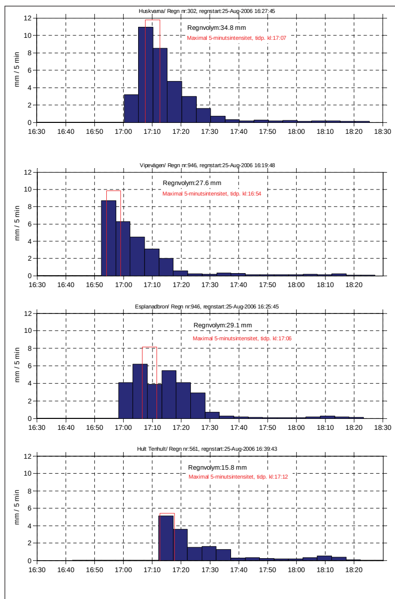
Figur 5-12 Exempel på nederbördsförlopp den 25/8 2006, registrerat i fyra nederbördsmätare i Jönköpings kommun.
