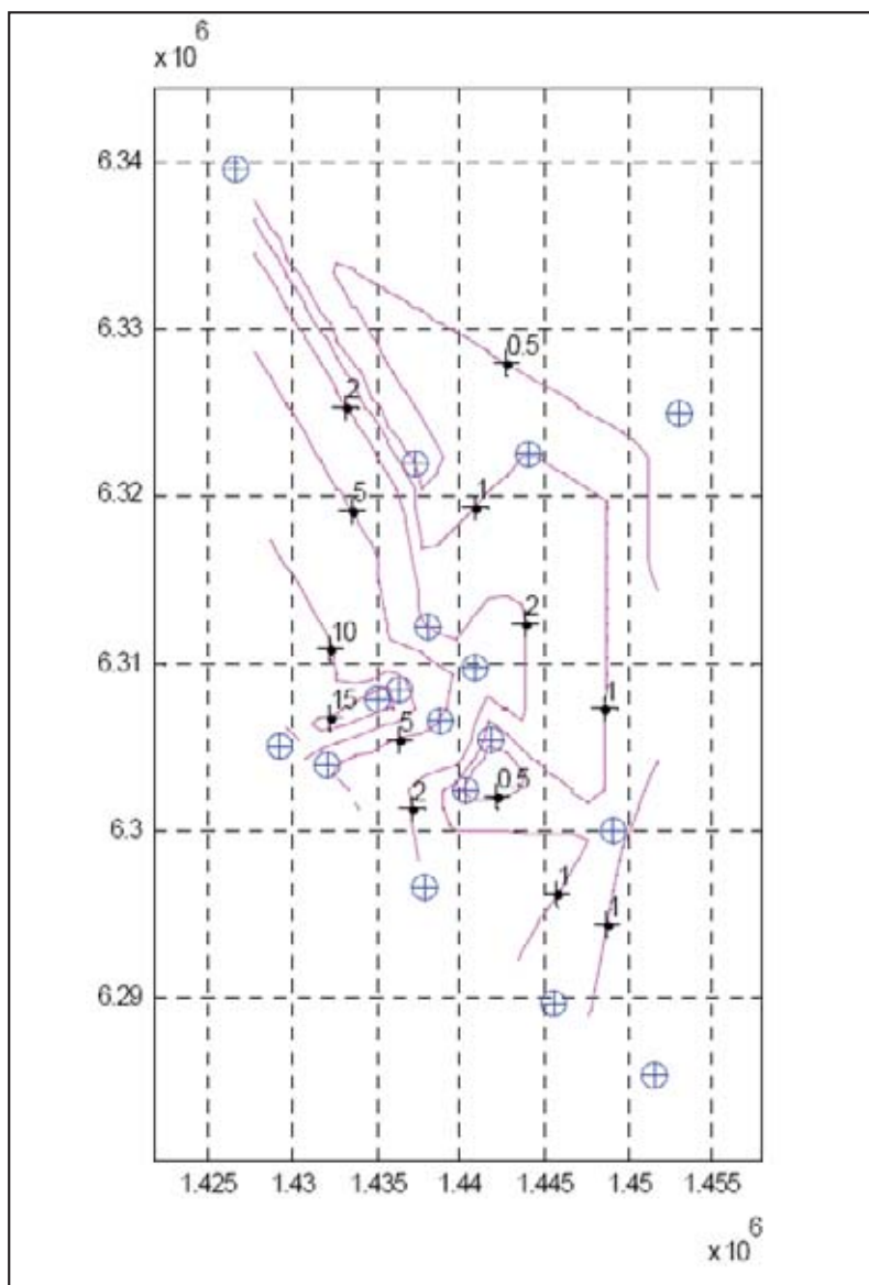
Figur 5-4 Regntillfälle den 30/9 2006 registrerat i 17 nederbördsrätare i Växjö kommun.
