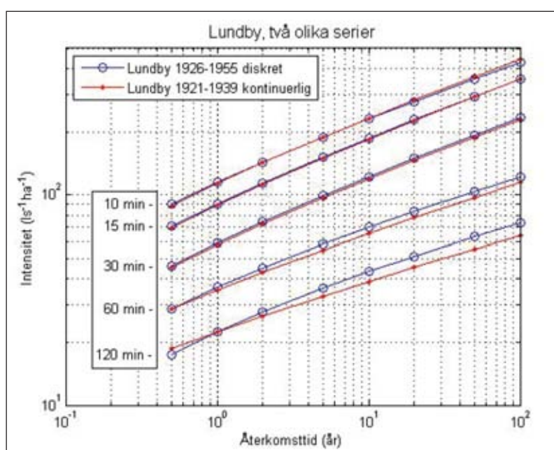
Figur 3-15 Jämförelse mellan blockregnstatistik för två olika regnserier från samma plats i Göteborg: Lundby 1926–1955 (regntillfällan) respektive Lundby 1921–1939 (kontinuerlig).
