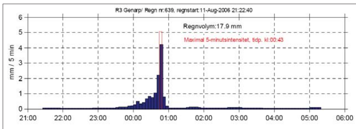
Figur 5-24 Registrerat nederbördsförlopp i Genarp, Lund den 11–12/8 2006.
