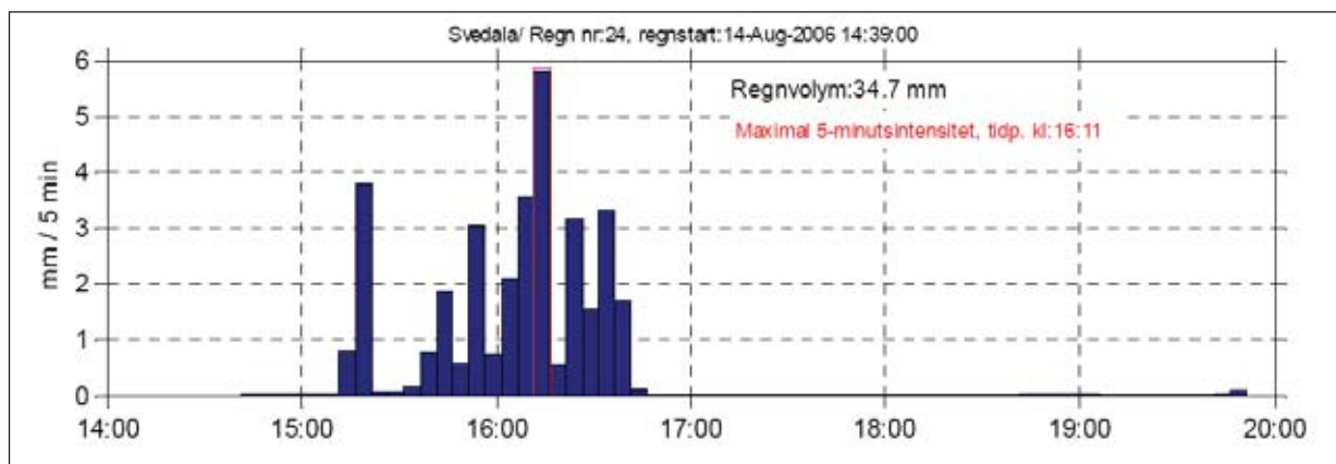
Figur 5-26 Registrerat nederbördsförlopp vid Svedala reningsverk den 14/8 2006.
