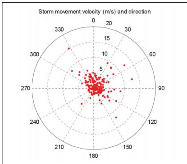
Figur 6-8 Hastighet (m/s) och rörelseriktning för 225 regntillfällen i Jönköping under perioden 1995–2006 bestämda utifrån regndata från 9 stationer. Regnurval: större än 4 mm, månaderna juni-september.
