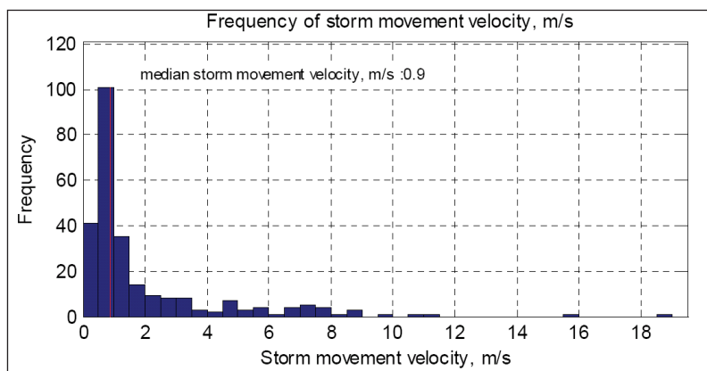
Figur 6-12 Fördelning av bedömd rörelsehastighet (antal per hastighetsintervall) för 285 regntillfällen i Växjö under perioden 2001–2007 bestämd utifrån regndata från 5 stationer. Regnурval: större än 4 mm, hela året.
