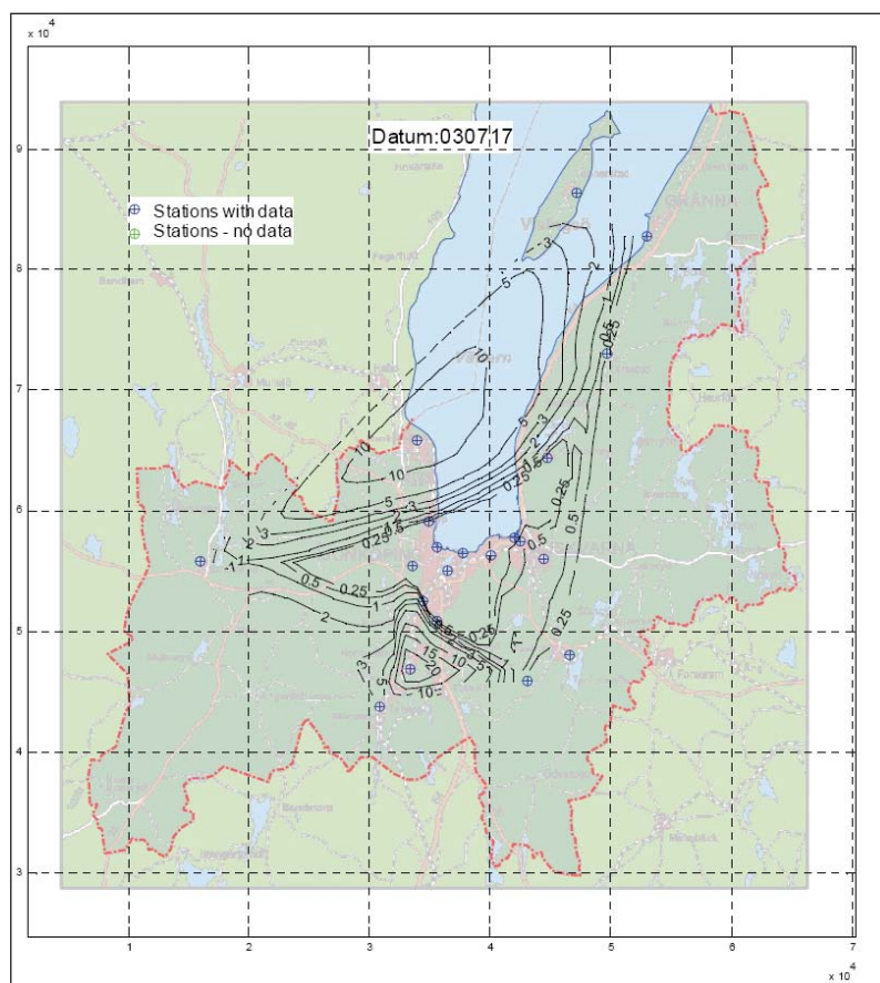
Figur 5-9 Regntillfälle den 17/7 2003 registrerat i 21 nederbördsrätmätare i Jönköpings kommun. Bilden visar nivålinjer för återkomsttid (år) – från 0,5 till 15 år, utvärderade som maximal återkomsttid för blockregnvaraktigheterna 5 min upp till 2 timmar för respektive stationsdata. Skalan på rutnätet i bilden är 10 x 10 km.
