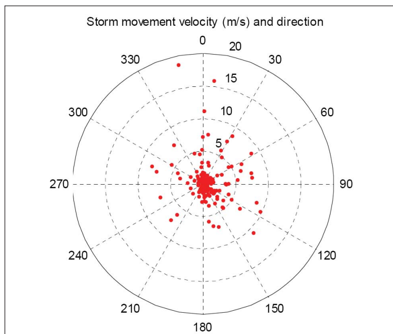
Figur 6-11 Hastighet (m/s) och rörelseriktning för 285 regntillfällen i Växjö under perioden 2001–2007 bestämda utifrån regndata från 5 stationer. Regnурval: större än 4 mm, hela året.
