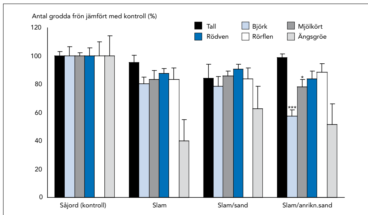
Figur 4-2 Groningsfrekvens av frön av 6 olika växtarter efter 3 veckor i rötslam, med eller utan inblandning av sand eller anrikningssand, jämfört med groning i såjord ( n=5\pm SE ). Stjärnor som är märkta med * är signifikant (*= p<0,05 ; **= p<0,01 , ***= p<0,001 ) lägre än kontrollen.
