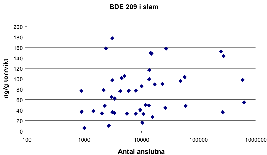
Fig. 10b. Halter av BDE 209 jämfört med storleken på ARV uttryckt som antal anslutna personekvivalenter efter att de 5 högsta värdena är borttagna.
