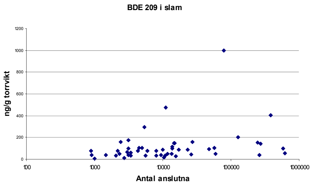
Fig. 10a. Halter av BDE 209 jämfört med storleken på ARV uttryckt som antal anslutna personekvivalenter.
