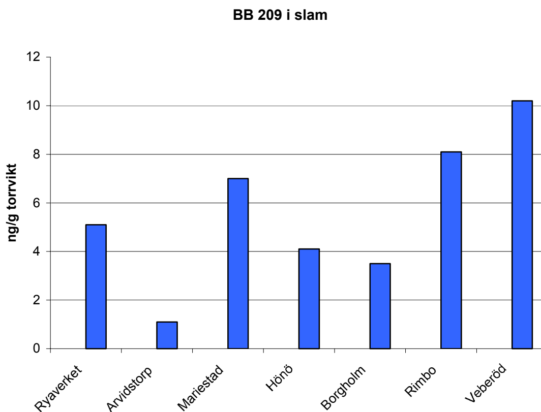
Fig. 16. Halter av BB 209 i slam från små, medelstora och stora ARV.
