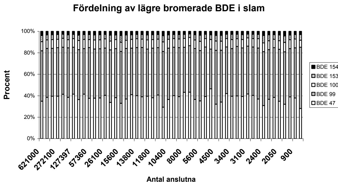
Fig. 9. Jämförelse av den procentuella fördelningen av BDE 47, 99, 100, 153 och 154 i alla slamprover fördelade efter antalet anslutna personekvivalenter.
