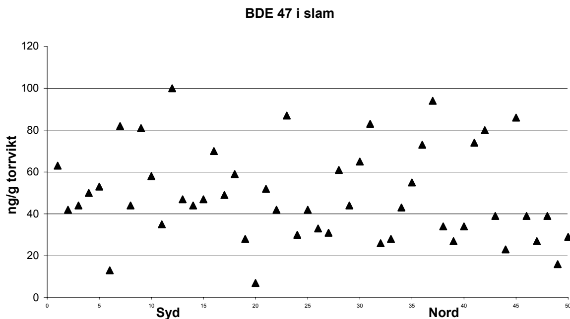
Fig. 20. Halter av BDE 47 jämfört med var i landet ARV ligger.
