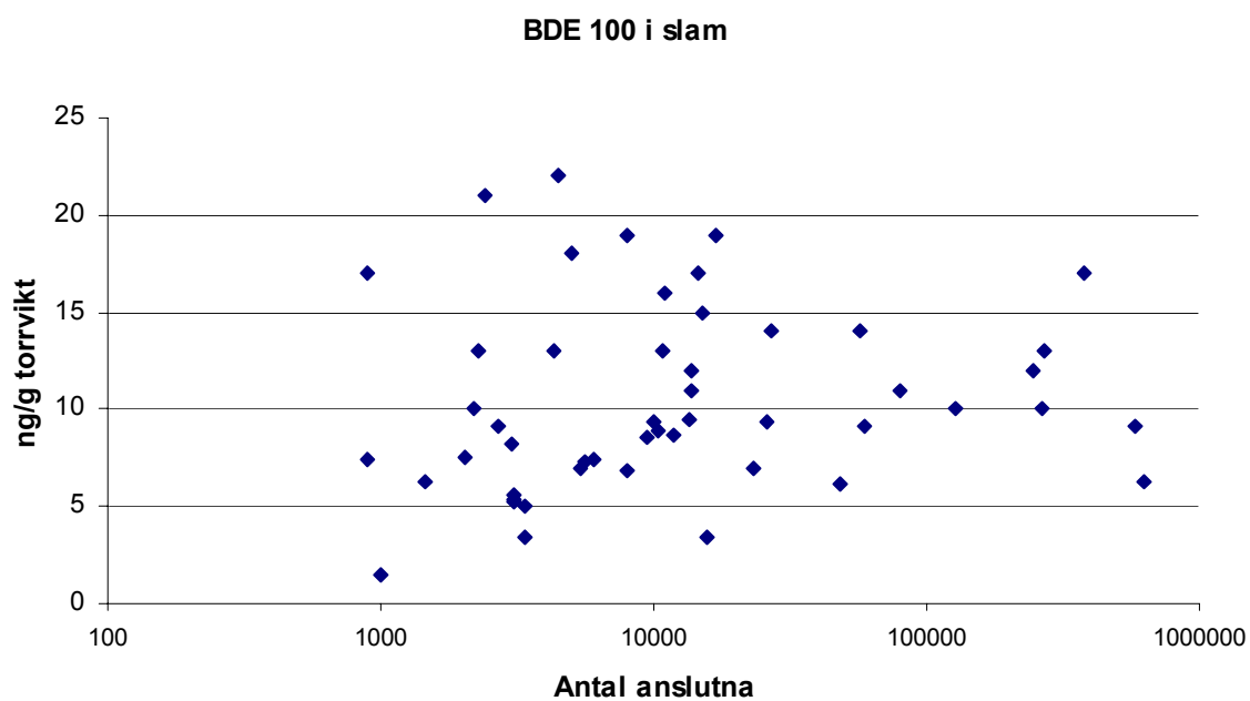
Fig. 3. Halter av BDE 100 jämfört med storleken på ARV uttryckt som antal anslutna personekvivalenter.
