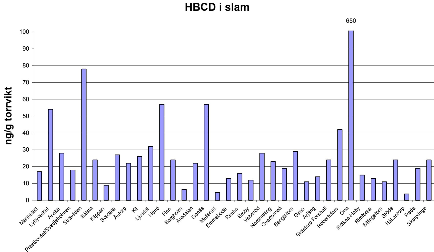
Fig. 15. Halter av HBCD i slam från små ARV
