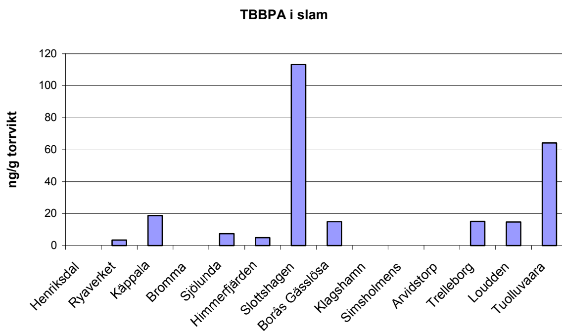
Fig. 18. Halter av TBBPA i slam från stora och medelstora ARV.
