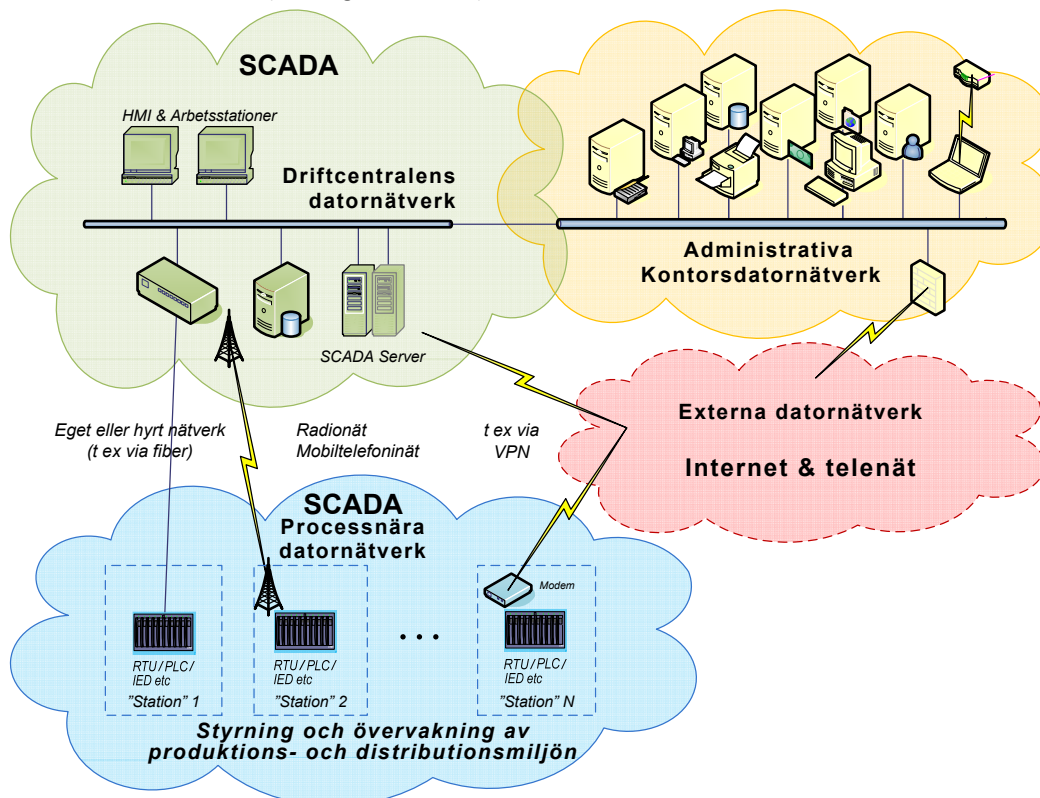
Figur 1. Referensmodell för att förtydliga terminologin som använts i denna enkät. Notera att termen SCADA används som ett samlingsbegrepp för all form av processkontrollstyrning som återfinns såväl i driftcentralens datornätverk (gröna molnet) som i produktions- och distributionsmiljön (blå molnet). Övriga områden som ofta interagerar med SCADA-system är datorsystem i det administrativa kontorsnätverket (gula molnet) samt datorsystem från underleverantörers tjänster som befinner sig på externa nätverk utanför er kontroll (röda molnet).
