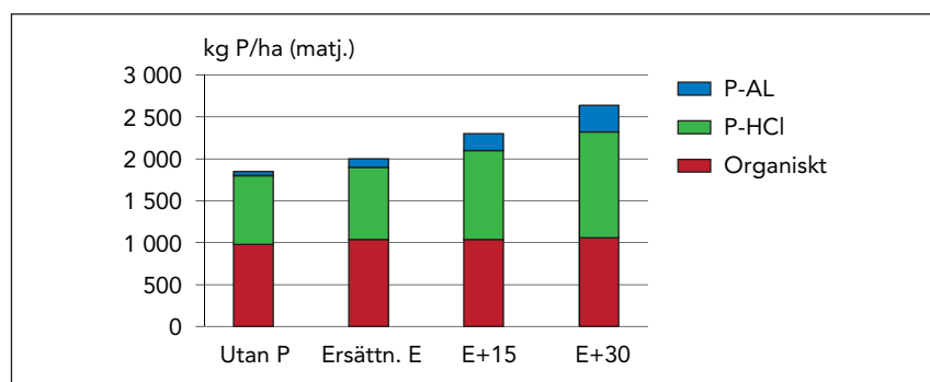
Figur 6-1 Bördighetsförsöket på Orup i Skåne (efter Olle Gunnarsson 1987). Fosforbehandlingarna är 0, ersättning för bortförsel (E), E+15 kg P per år och E+30.
