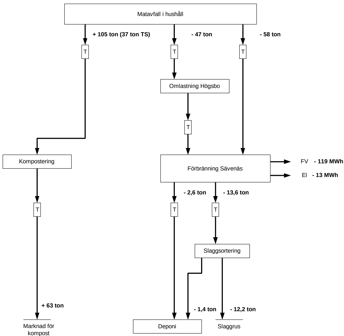
Figur B6.2. Förändring av årliga avfalls- och energiflöden i Göteborg vid behandling av matavfall från 1000 hushåll genom central kompostering istället för förbränning. Rutor markerade med bokstaven T symboliserar lastbilstransport.
