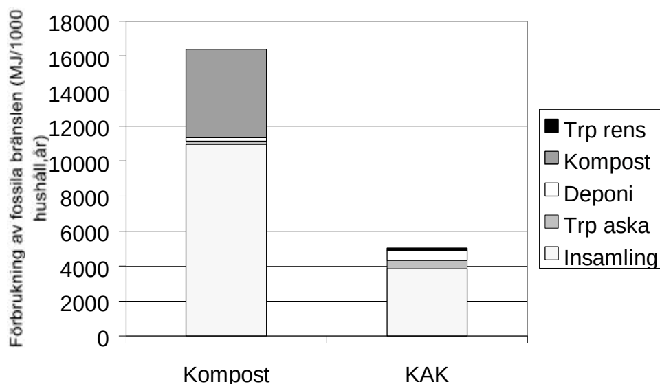
Figur 3.3 Förbrukning av fossila bränslen. (Kompost = det renodlade komposteringssystemet, KAK = systemet med köksavfallsskvarnar, MJ är ca 0.28 kWh)
