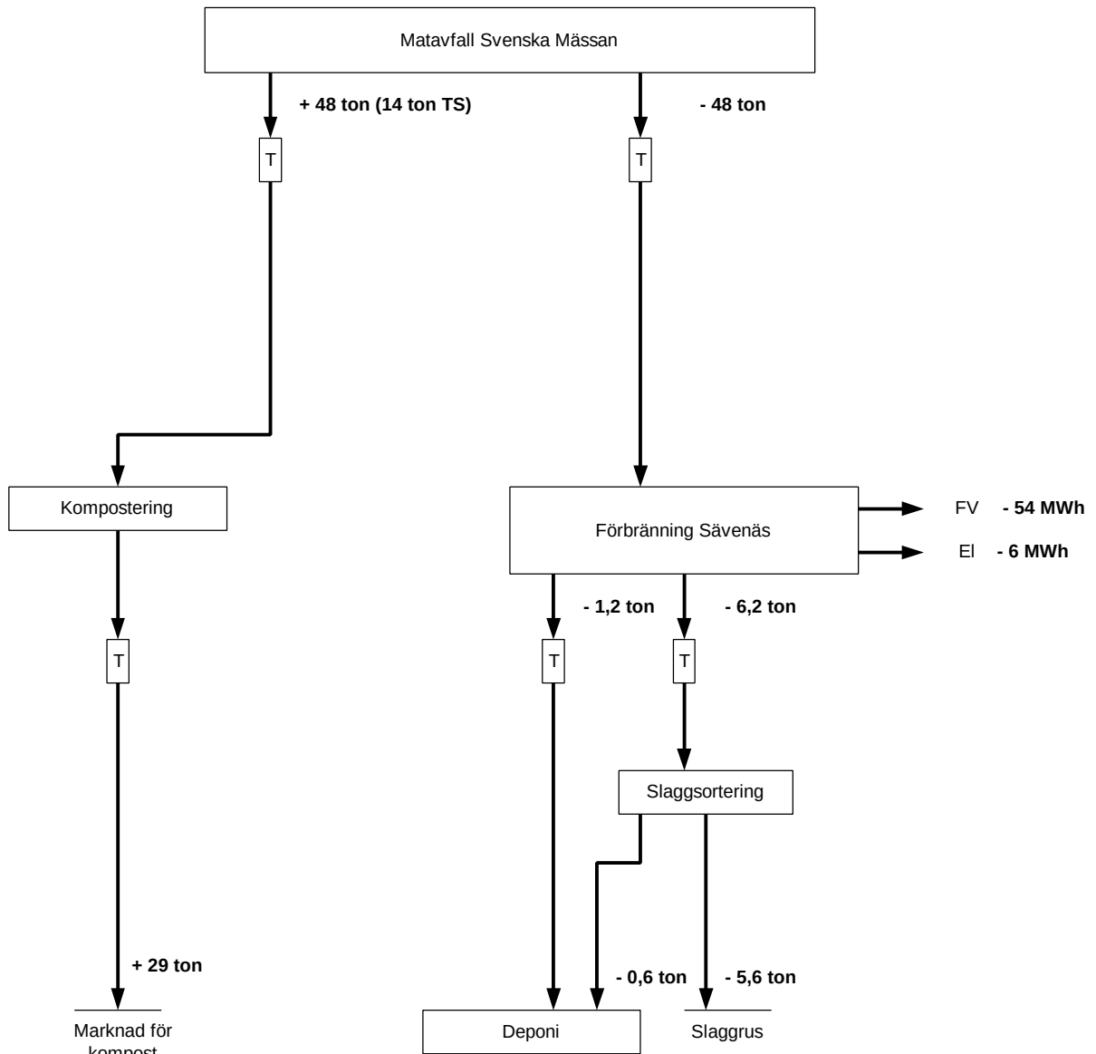
Figur B6.4. Förändring av årliga avfalls- och energiflöden i Göteborg vid behandling av matavfall från Svenska Mässan genom central kompostering istället för förbränning. Rutor markerade med bokstaven T symboliserar lastbilstransport.
