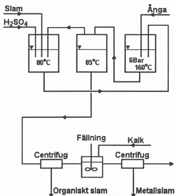
Figur 6. Slambehandling med termisk hydrolys. (Karlsson och Göransson 1992)
